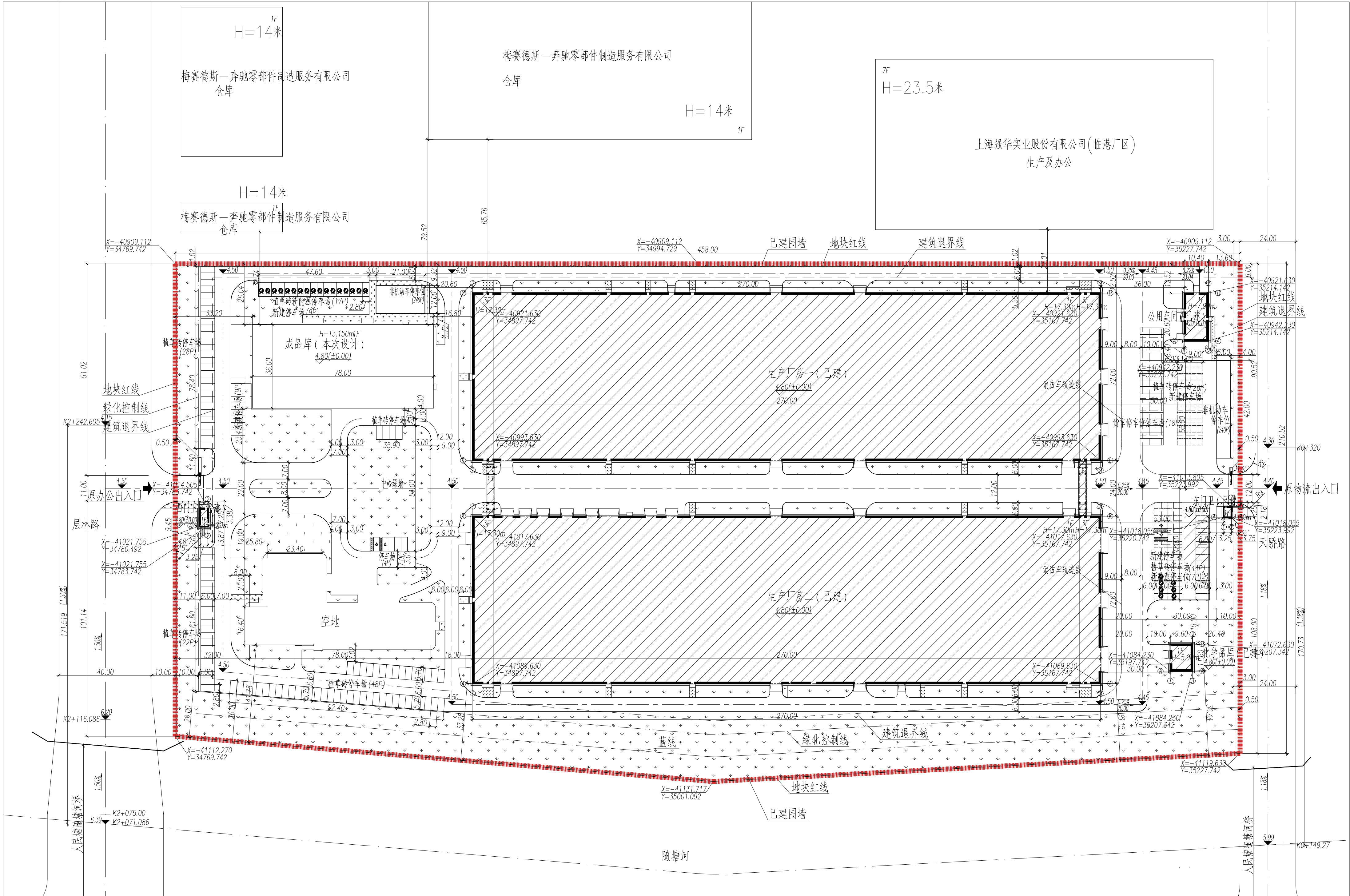
总平面布置图
